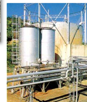
消化ガス用乾式脱硫装置
